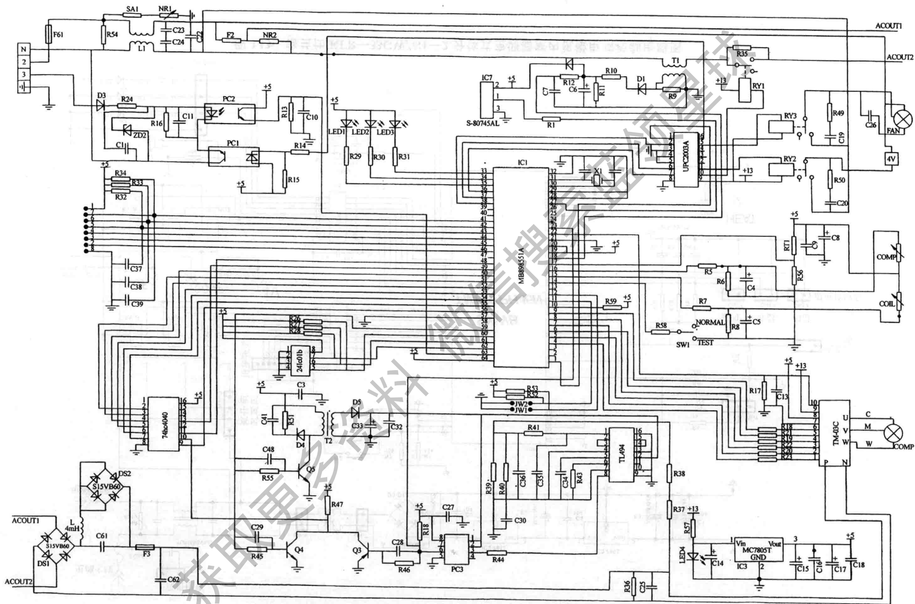
图 142 格兰仕 KFR—28GW 变频分体式空调器室外机电脑控制电路图
