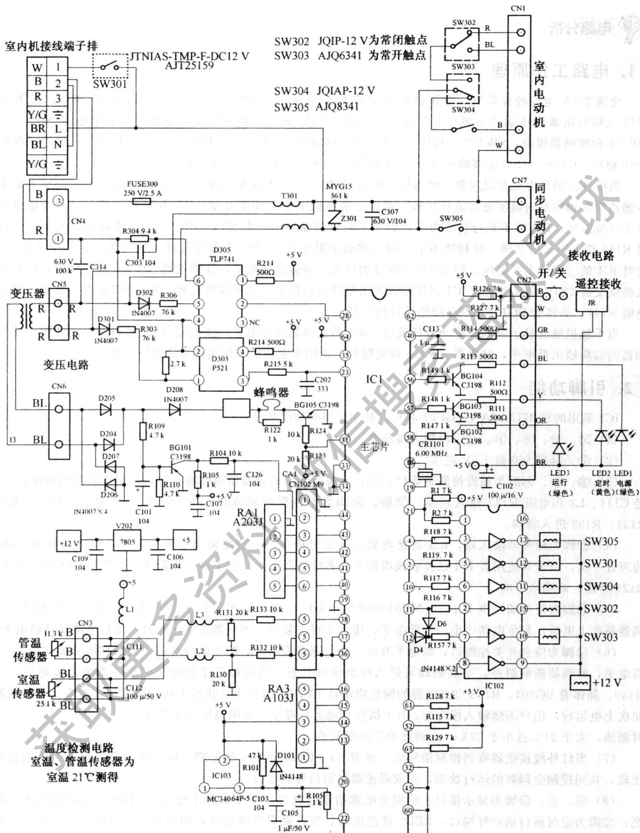
图 40 海尔 KFR—50LW/BPF 变频柜式金元帅空调器室内机微电脑控制电路图
