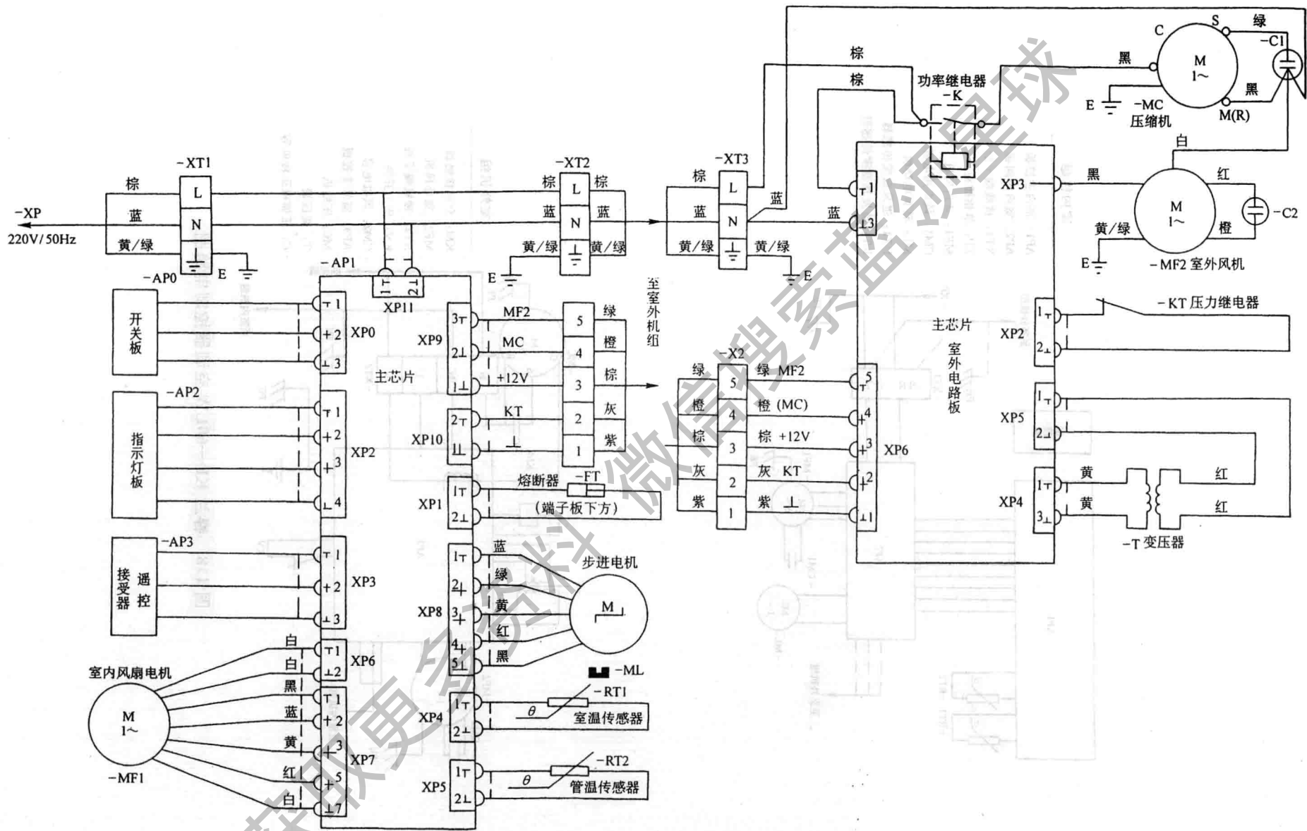
图 117 春兰 KF-40GW 型分体式空调器控制电路图
