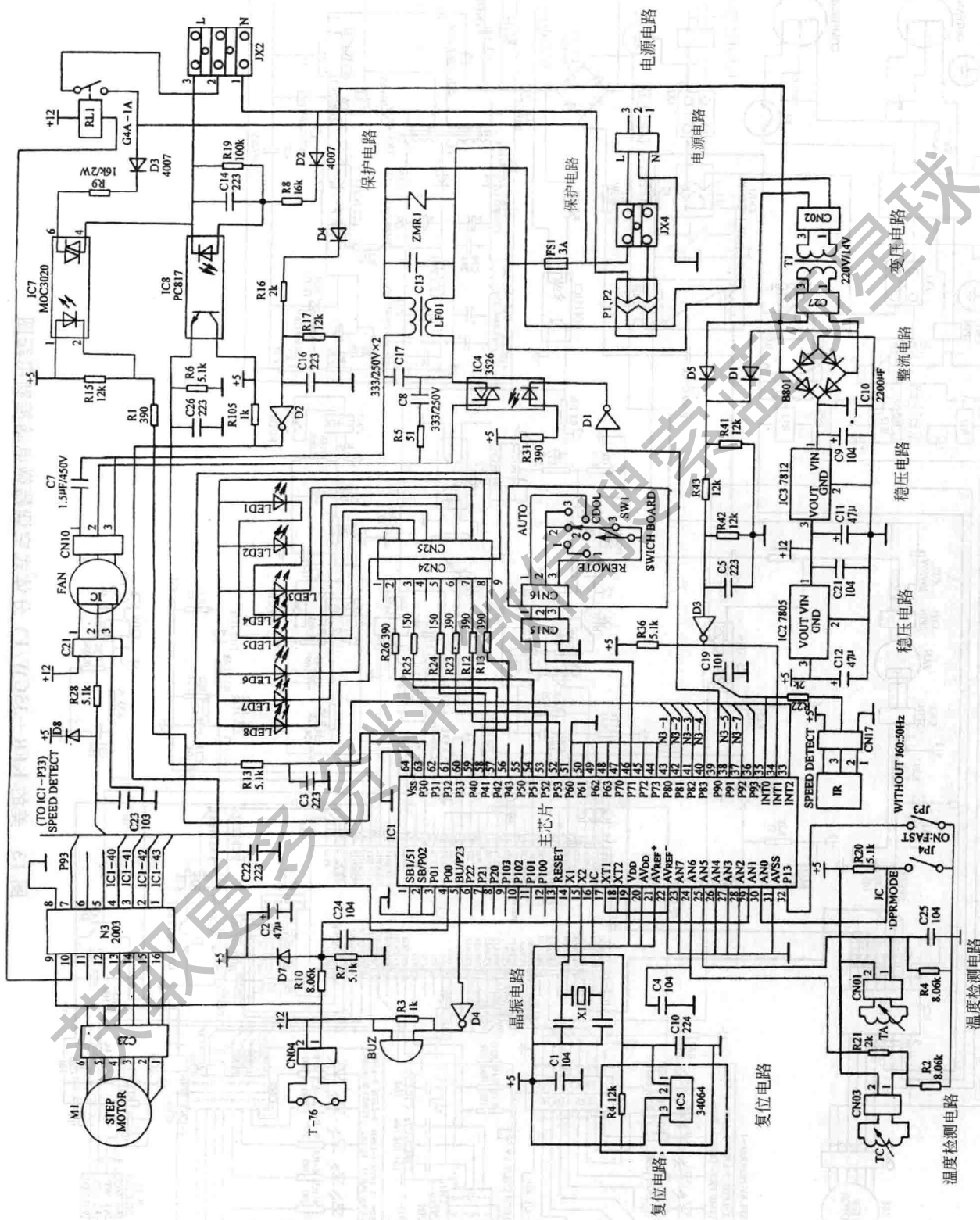
图 14 美的 KFR-36GW/BPY 变频分体式空调器室内机微电脑控制电路图
