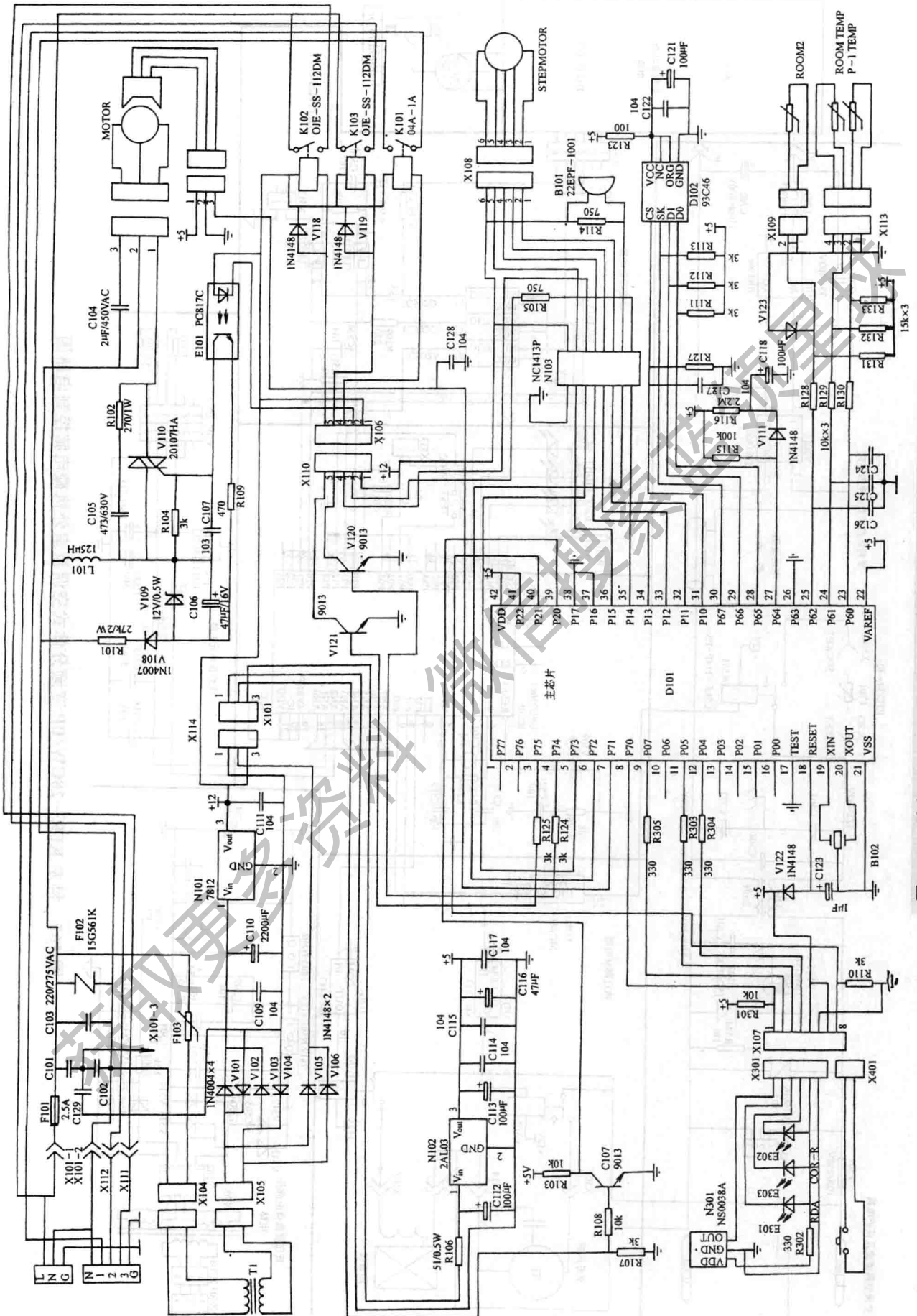
图 164 科龙 KFR-42GW/C2 空调器室内机微电脑控制电路图
