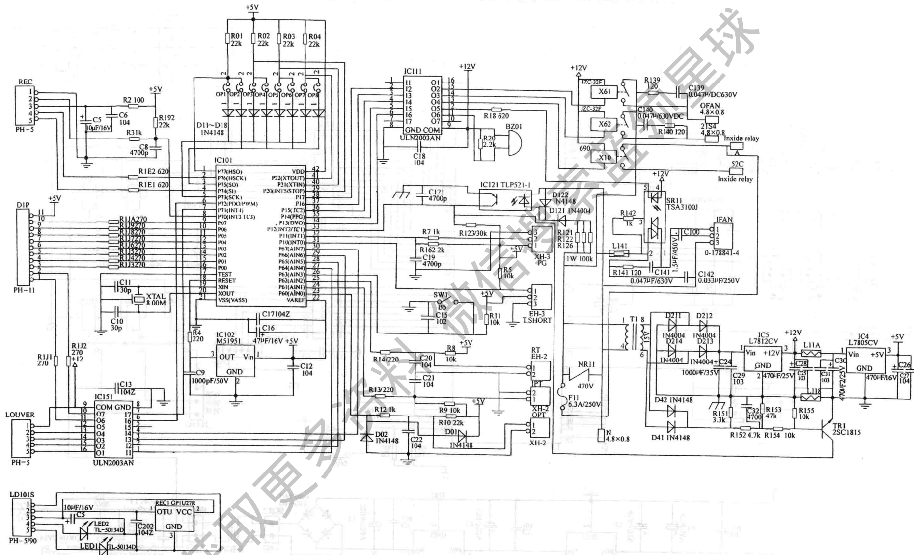
图 147 格兰仕 KFR-25GW/A1 分体式空调器室内机微电脑控制电路图
