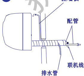
图16 挂墙板
