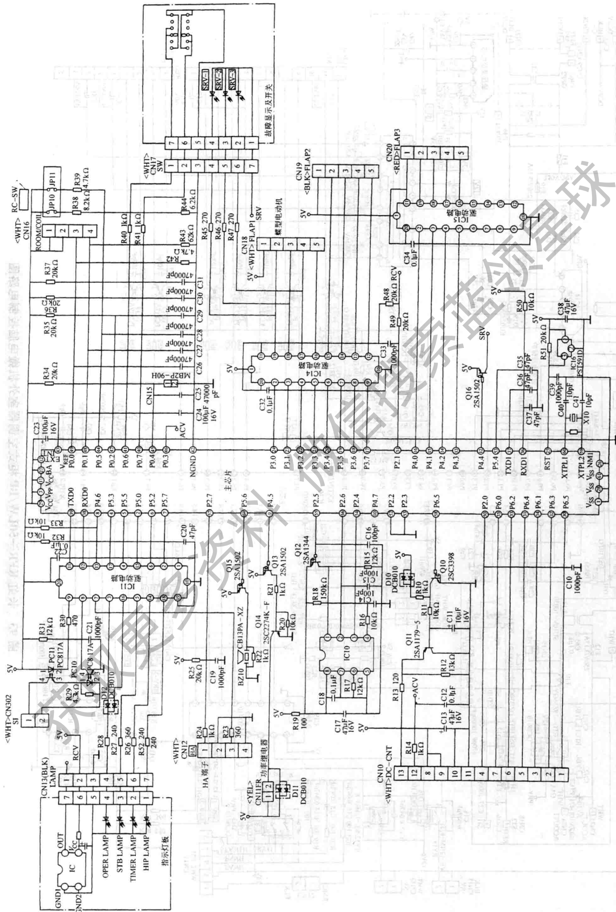
图 94 长虹 KFR—50LW/BP 柜式空调器室外机微电脑控制电路图
