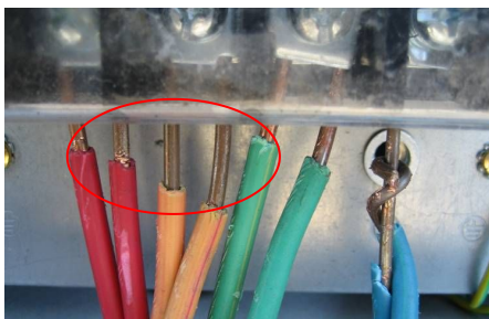
电源线裸露部分太多，存在安全隐患（错误）
