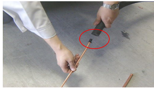
铜管封口后，再套保温管（正确）
