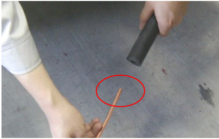
铜管套保温管的时候没有封口，导致杂物入管内（错误）
